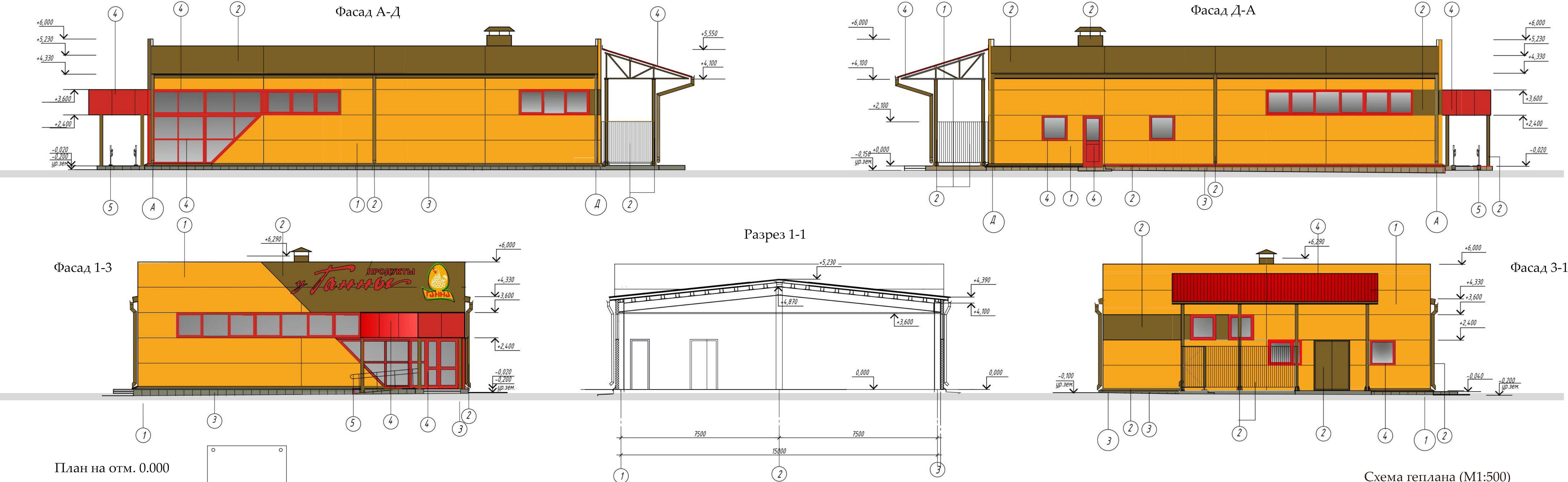
Схема генплана (М1:500)
